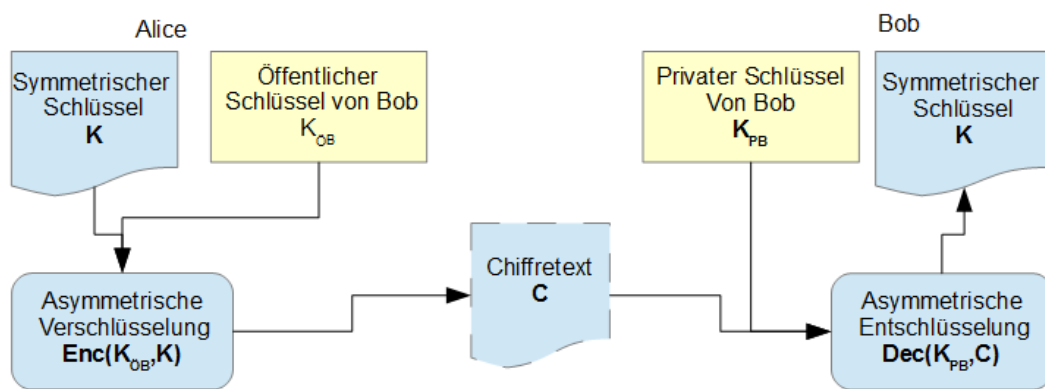
Abbildung 4: Schlüsselaustausch mittels asymmetrischer Verschlüsselung
