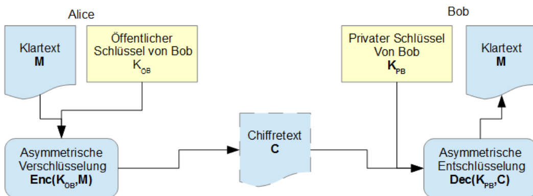
Abbildung 2: Asymmetrische Verschlüsselung 1
