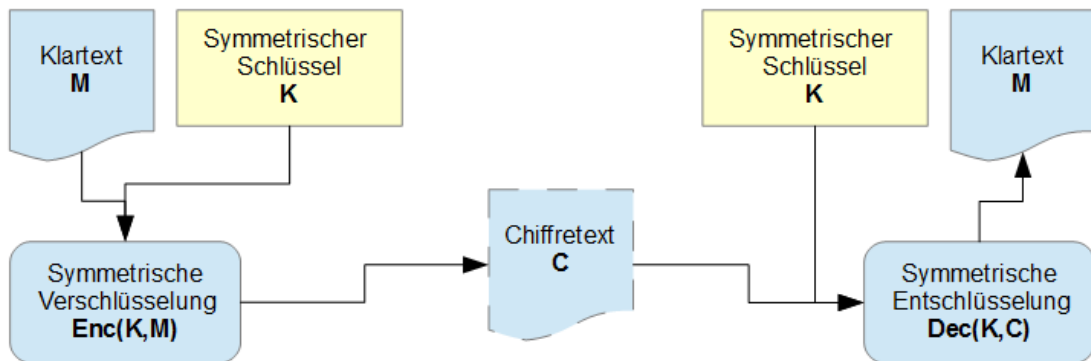
Abbildung 1: Symmetrische Verschlüsselung
