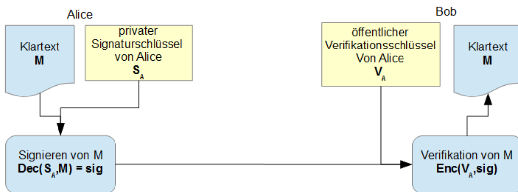
Abbildung 5: Signatur
