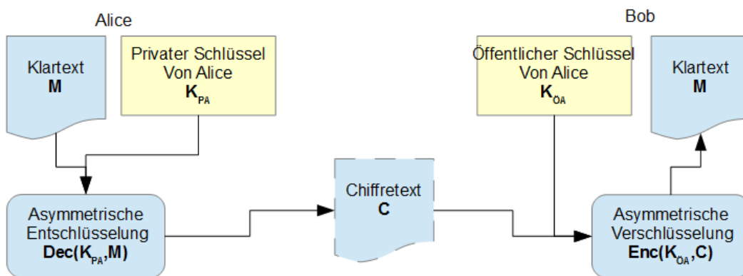
Abbildung 3: Asymmetrische Verschlüsselung 2
