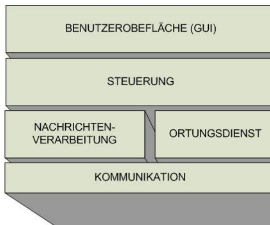
Abbildung 6.8: Strukturierung des Clients
