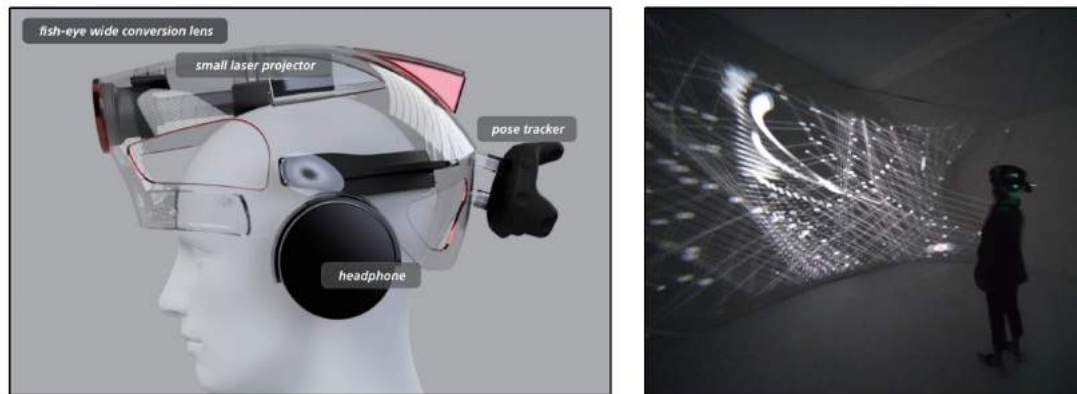
Abbildung 2.9: Head-Mounted Projektor Display „HeadLight“, Quelle: Kasahara [11]
