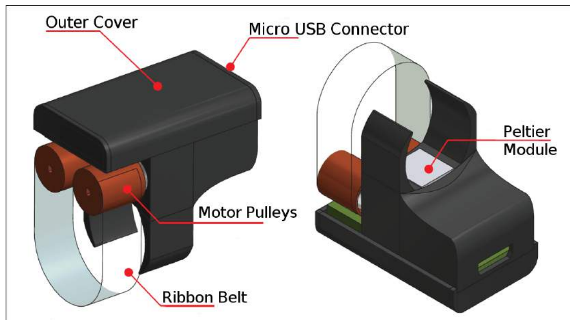
Abbildung 2.10: „Altered Touch“, Quelle: Takaki u. a. [27], leicht abgeändert
