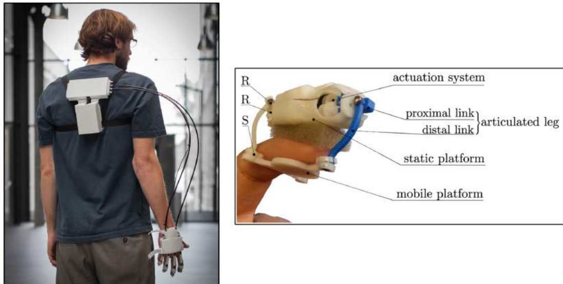
Abbildung 2.11: „3RRS wearable fingertip cutaneous device“, Quelle: Chinello u. a. [3]
