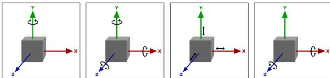
Abbildung 2.4: a) Magnetometer Messung, b) Messung von drei Gyroskopen, c) Positionsmessungen von drei Beschleunigungsmessern, d) Rotationsmessung von zwei Beschleunigungsmessern Quelle: Nadia Hintze 2018
