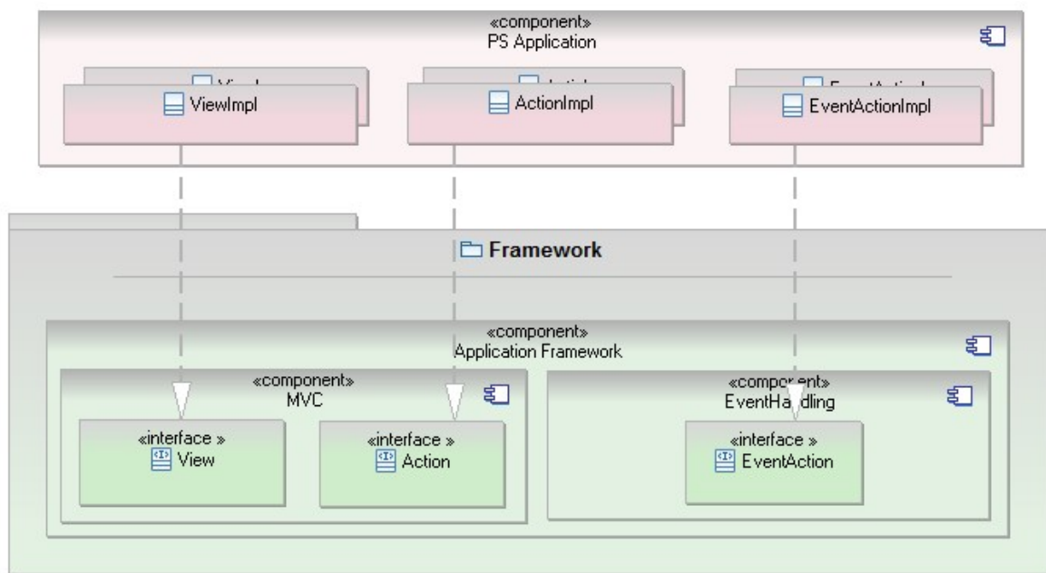
Abbildung 5.2: Model-View-Controller-Komponente
