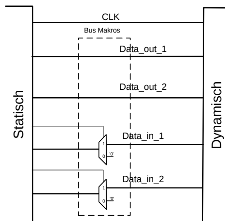
Abb. 3: Kommunikation zwischen statischem und dynamischen Modul über Bus Makros
