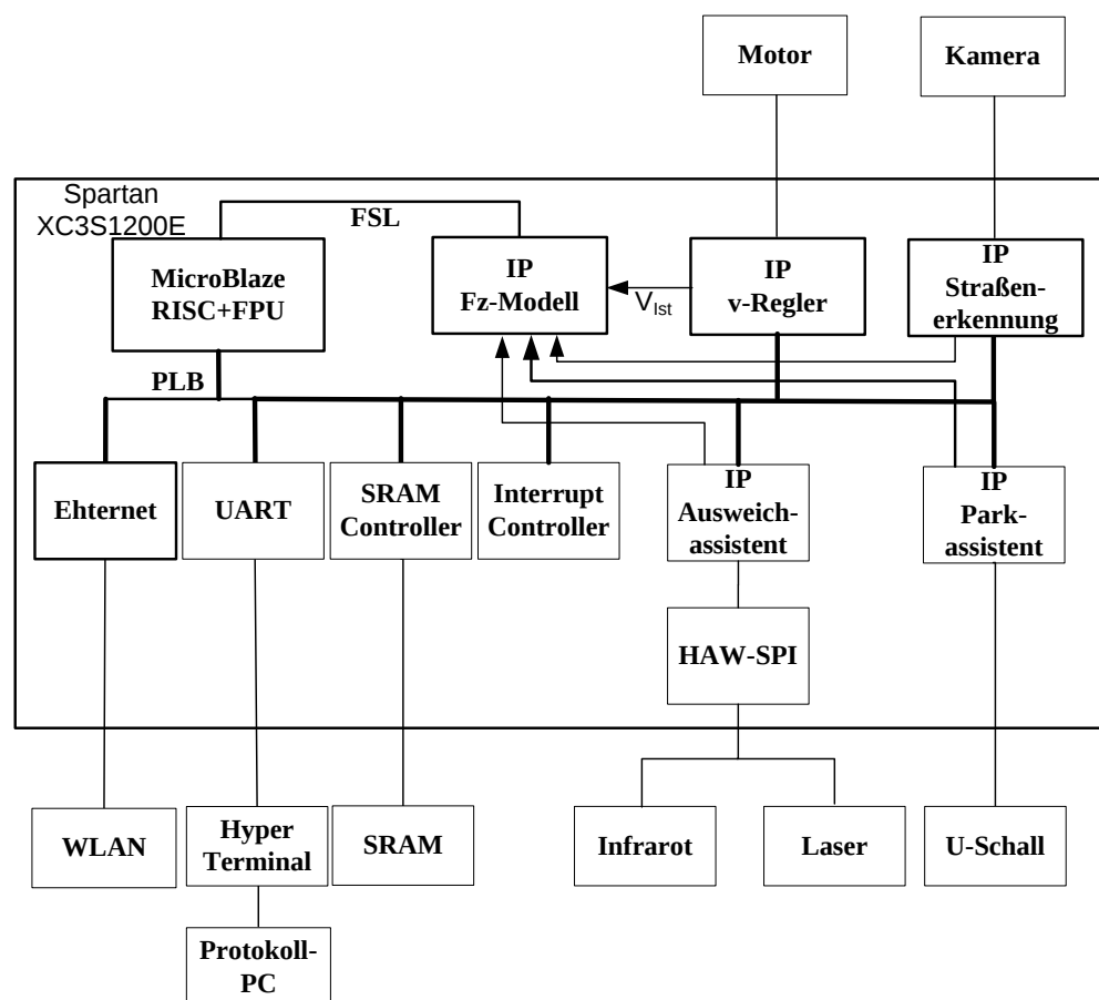
Abb. 1: FPGA-basierte SOC-Steuerplattform für ein autonomes Fahrzeug sowie Bildverarbeitungs- und Sensorauswertungseinheiten.
