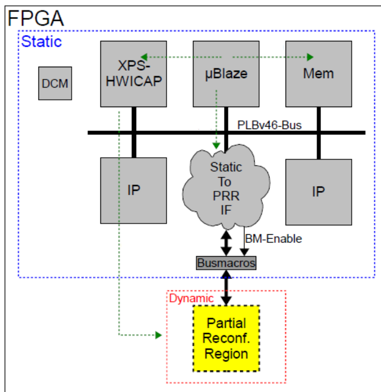
Abb. 4: Modularer Aufbau des PR-Testsystems mit Petalinux [Mamegani (2010)]
