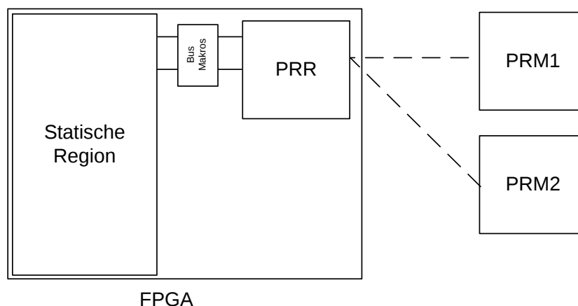
Abb. 2: System mit Statischem- und Rekonfigurationsblock
